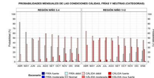
Figura 2. Probabilidades mensuales de las categorías de las condiciones cálidas, frías y neutras según el ICEN para el Pacífico central (región Niño 3.4, barras de la izquierda) y probabilidades según el ICEN para el extremo del Pacífico oriental (región Niño 1+2, que abarca la zona norte y centro del mar peruano, barras de la derecha) de abril de 2026 a enero de 2027, estimadas por el ENFEN.
