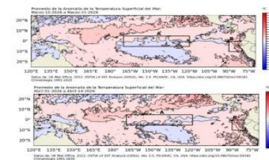
Figura 1. Distribución de las anomalías de la Temperatura Superficial del Mar (TSM) en el Pacífico tropical y ubicación de las regiones Niño 3.4, en el Pacífico central, y Niño 1+2, frente a la costa peruana, delimitadas con recuadros de color negro. Arriba: promedio de las anomalías de la TSM para el periodo 15-31 de marzo de 2026. Abajo: promedio de las anomalías de la TSM para el periodo 1 - 14 de abril de 2026. Fuente: OSTIA.
